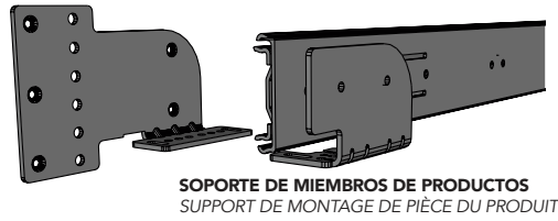
FIGURE 4.1 SOPORTE DE MONTAJE LATERAL / SUPPORT DE MONTAGE LATÉRAL
